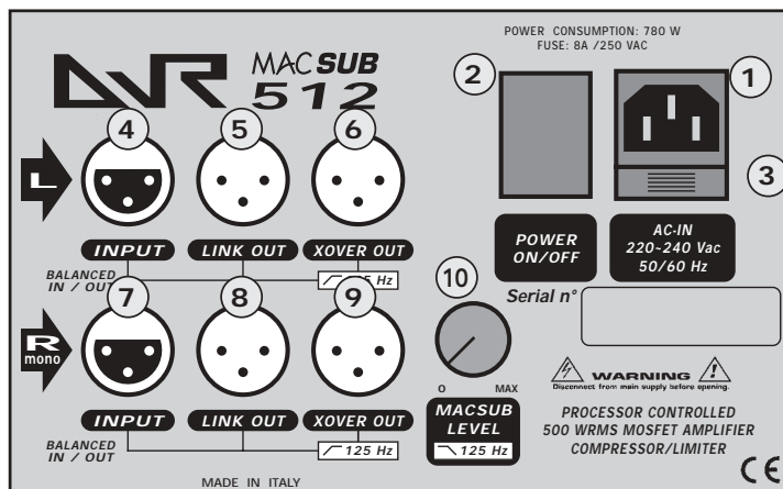
Pannello posteriore
